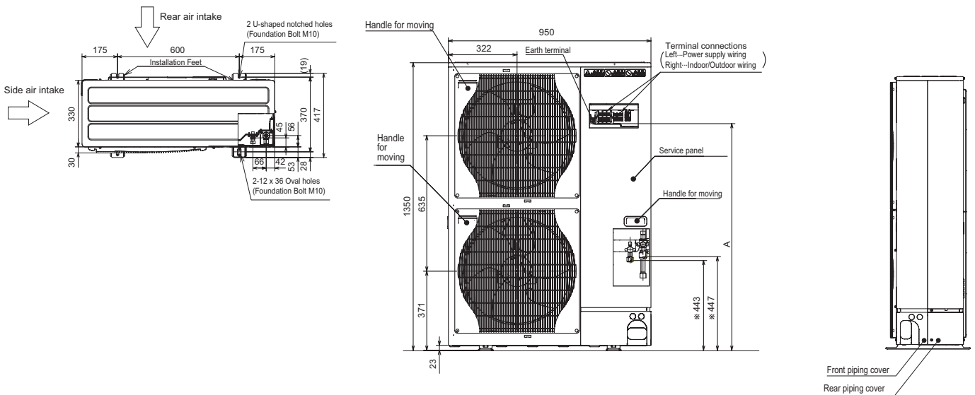
Venkovní jednotky Zubadan Inverter new generation, PUHZ-SHW112/140VHA-A/YHA-A
