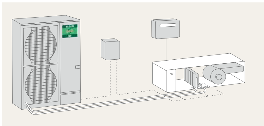
Použití rozhraní PAC-IF013B-E se vzduchotechnickou jednotkou
