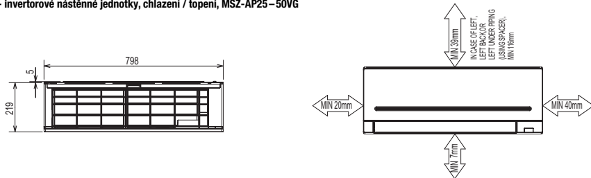
MSZ - invertorové nástěnné jednotky, chlazení / topení, MSZ-AP25-50VG
