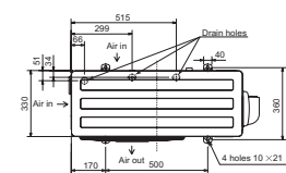
MUZ - invertorové venkovní jednotky, chlazení / topení, MUZ-EF50VG
