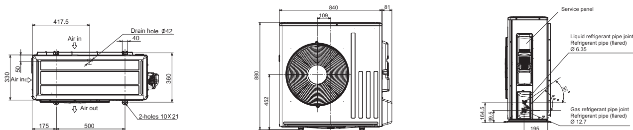
SUZ - invertorové venkovní jednotky, chlazení / topení SUZ-M60/71VA
