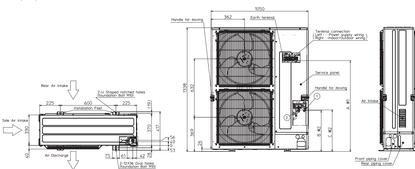
Venkovní jednotky Power Inverter, PUZ-ZM/PUHZ-ZRP100-140 YKA
