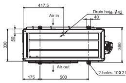
MUZ - invertorové venkovní jednotky, chlazení / topení, MUZ-AP20-42VG
