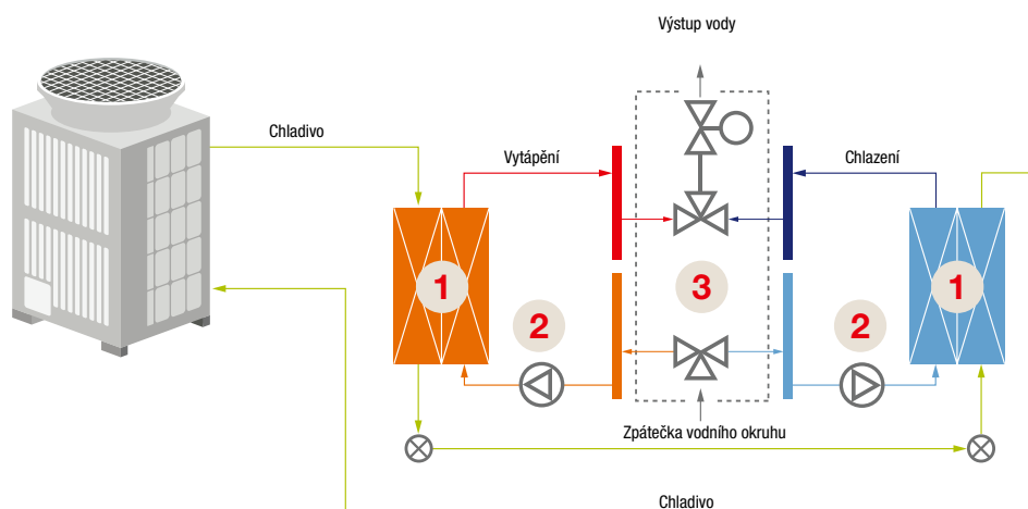
Schéma HBC controlleru
