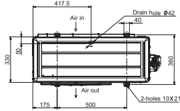
MUZ - invertorové venkovní jednotky, chlazení / topení, MUZ-AP50VG
